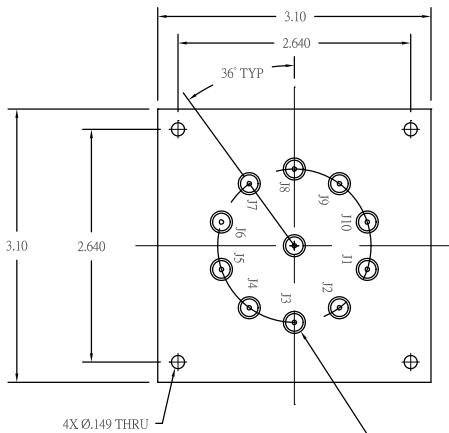
4X Ø.149 THRU
